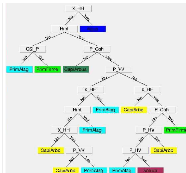
Figura 1. Árvore de decisões para atributos selecionados pelo Weka.
